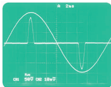
PCR-W/W 2 シリーズの出力波形 (50V/div, 5A/div)
